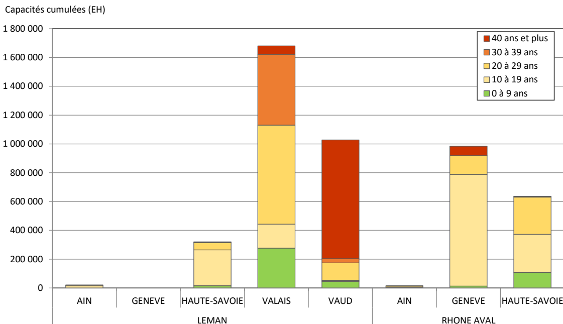
Figure 3 : Capacités théoriques d'épuration dans chaque secteur du territoire en fonction de l'âge des équipements en 2021 ou de la dernière rénovation de la filière « eau » (EH)
