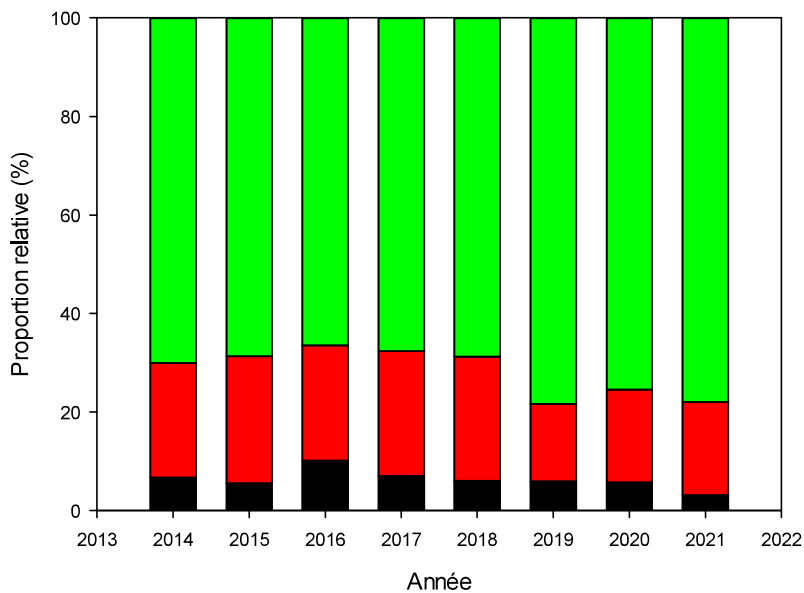
Figure 6 : Evolution de la proportion (en %) de biomasse des compartiments pico-, nano- et microphytoplanctoniques dans le Léman à la station SHL2 pour la période 2014-2021 entre 0 et 18 m.
