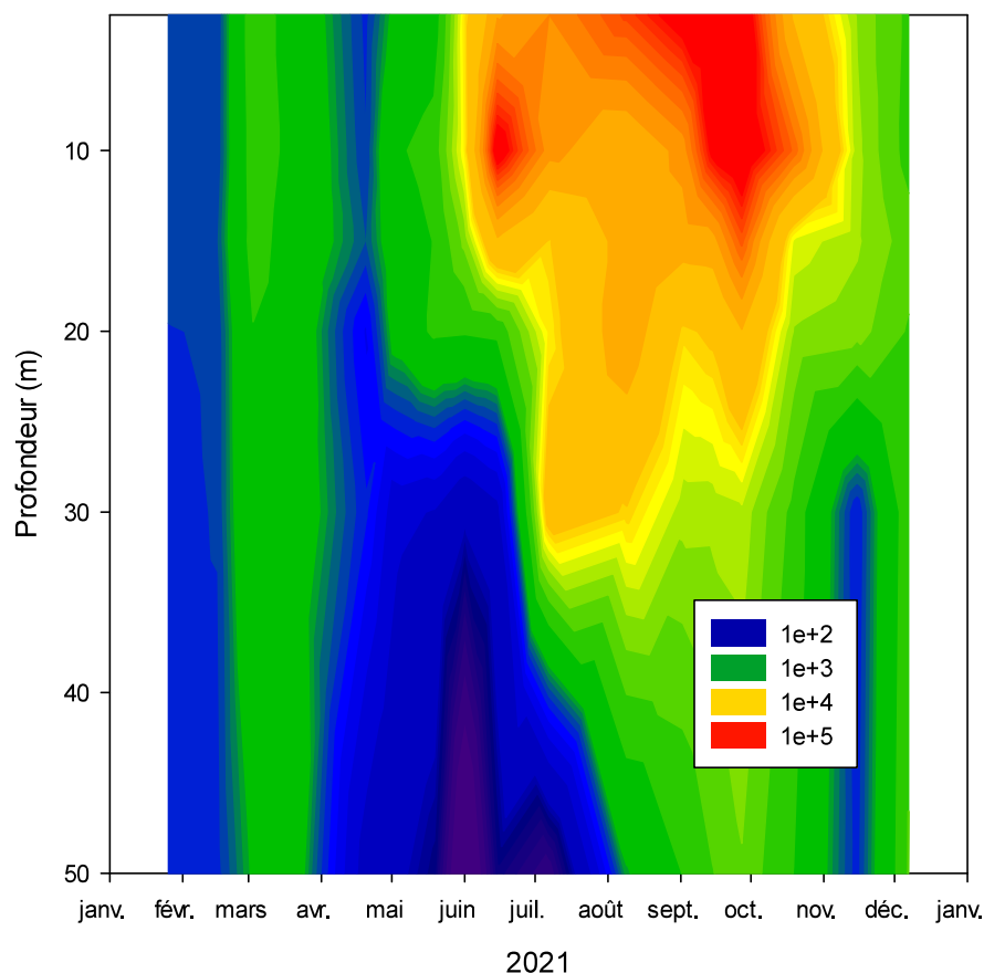
Figure 2 : Distribution et dynamique des picocyanobactéries (en cellules / mL) en 2021 entre la surface et 50 m de profondeur dans le Léman à la station SHL2. L'échelle proposée est la suivante: 1e+2= 100 ; 1e+3= 1000 ; etc.
