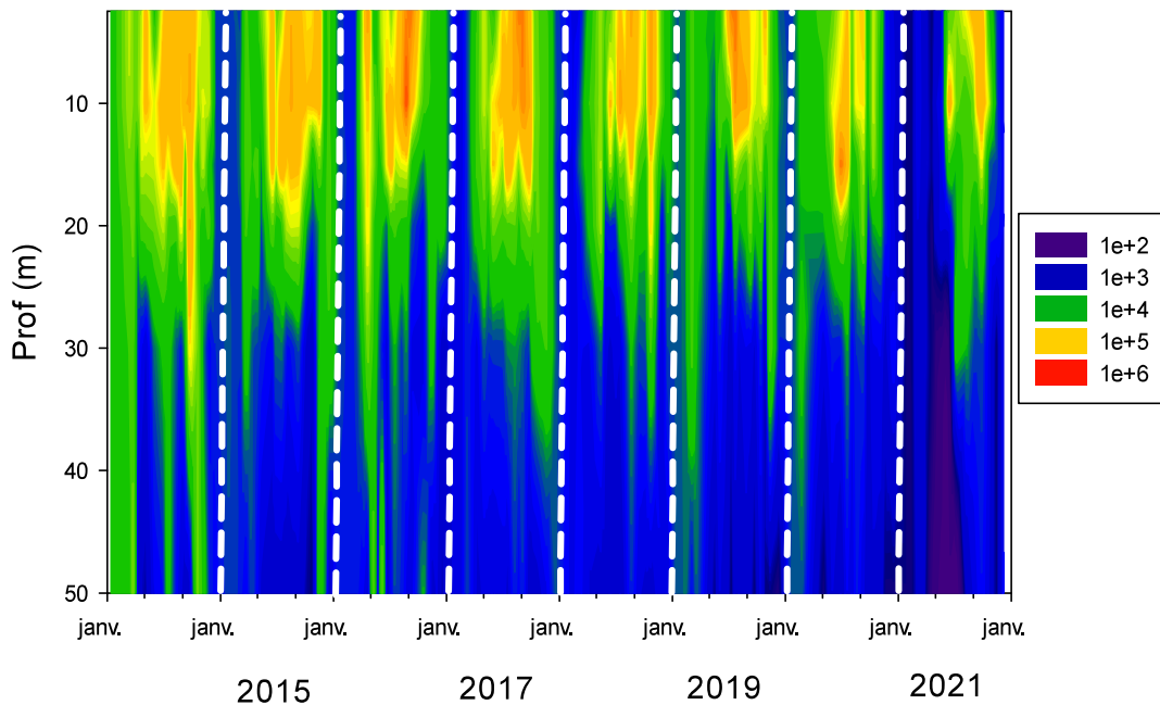
Figure 5 : Evolution des concentrations de picocyanobactéries entre 2.5 et 50 m, de 2014 à 2021 inclus, dans le Léman à la station SHL2.
