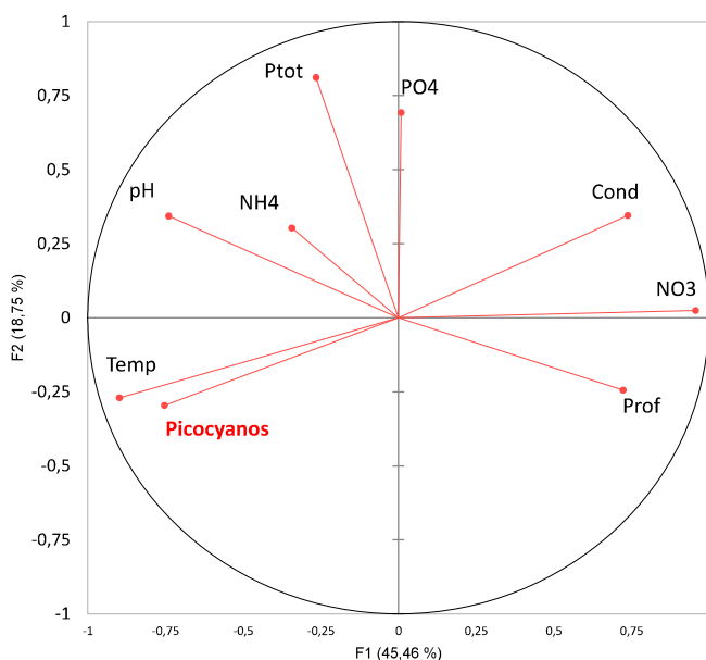
Figure 3 : Analyse en composantes principales (ACP) effectuée avec quelques paramètres sur l'ensemble de l'année 2020, dans le Léman, à la station SHL2. La variance totale expliquée est de 64,2%.
