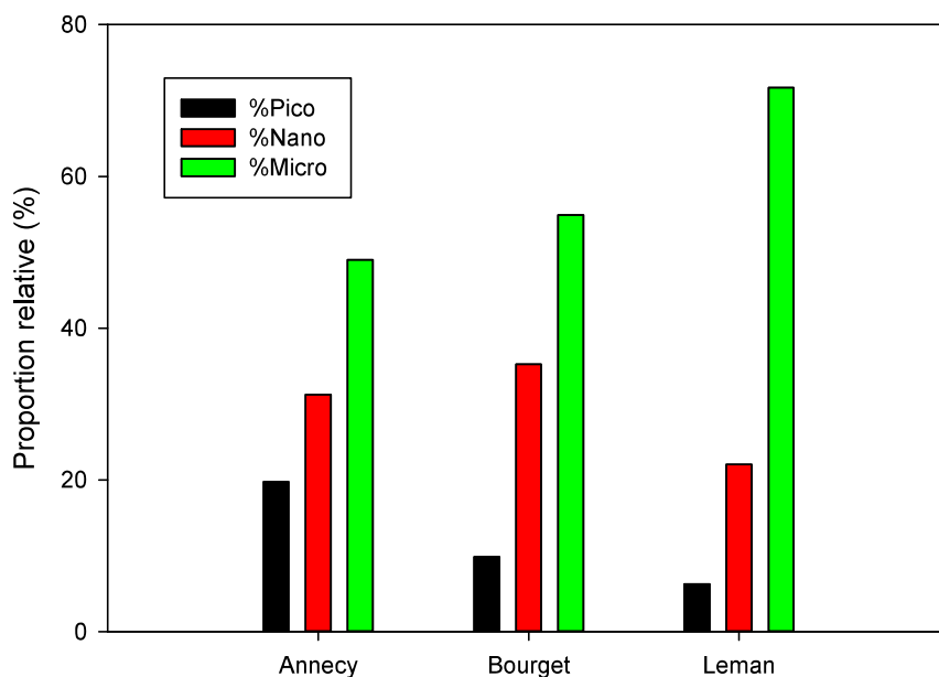
Figure 7 : Evolution de la proportion (en %) de biomasse des compartiments pico-, nano- et microphytoplanctoniques dans les lacs Léman, d'Annecy et du Bourget pour la période 2014-2021.
