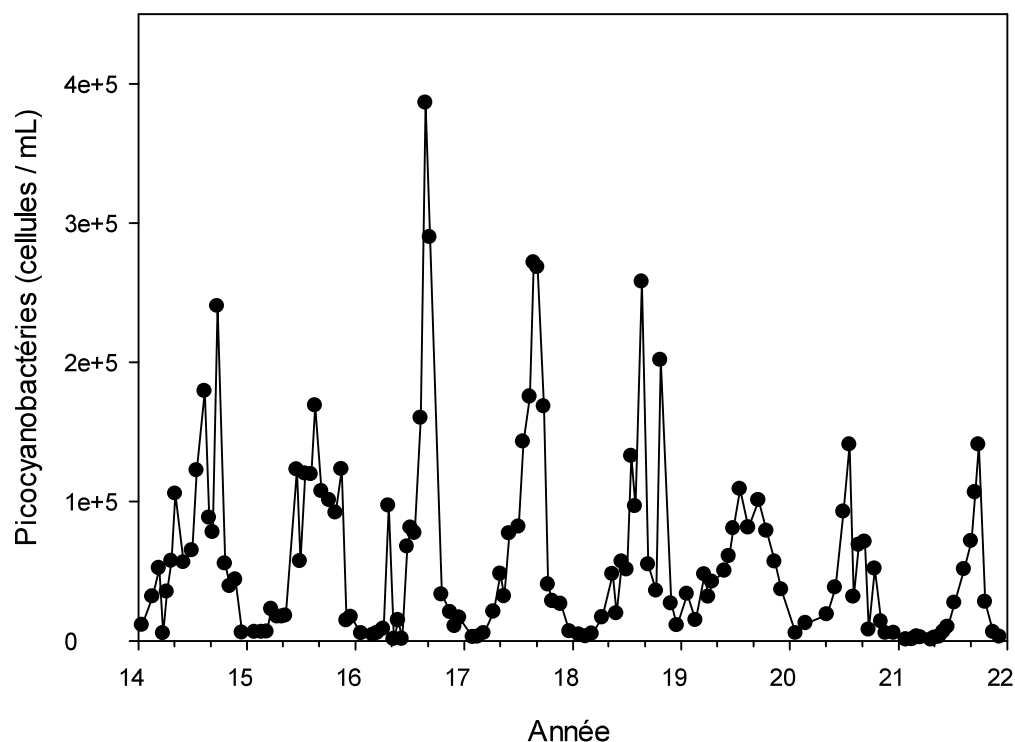
Figure 4 : Evolution des concentrations moyennes de picocyanobactéries (en cellules/mL) entre 2.5 et 20 m de 2014 à 2021 inclus, dans le Léman, à la station SHL2.
