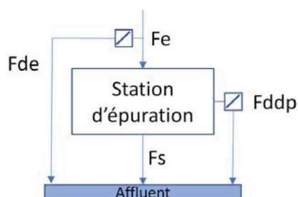
Figure 3 : Schéma des flux d'une station d'épuration
