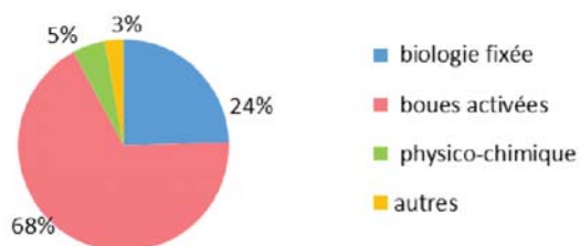
Figure 1 : Répartition de la capacité épuratoire totale des STEP du territoire suivant les procédés d'épuration Figure 1 : Distribution of the territory's WWTPs total treatment capacity according to the treatment processes used
