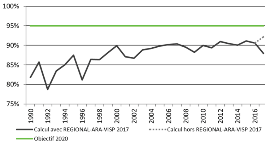
Figure 6 : Évolution entre 1990 et 2017 du rendement d'épuration du phosphore total sur les eaux traitées des STEP du bassin du Léman (en vert, objectif 2020 du Plan d'action)
